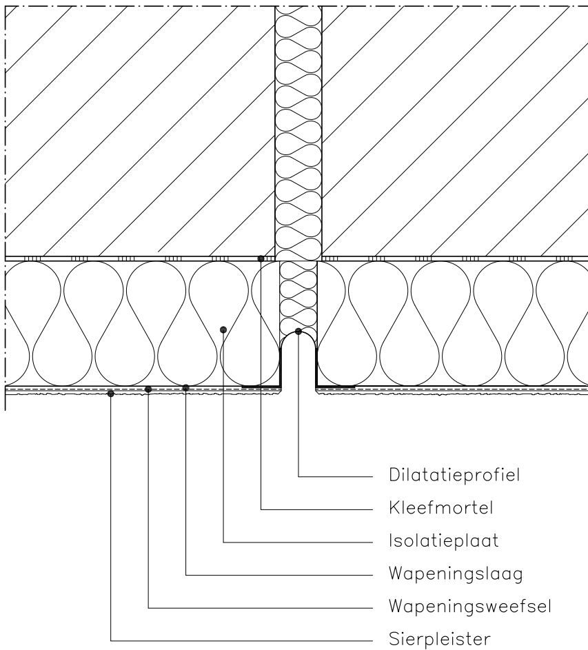
Afb. 18: Uitzettingsvoeg in het vlak
