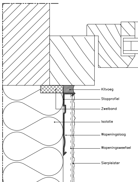
zwelband gecombineerd met kitvoeg
