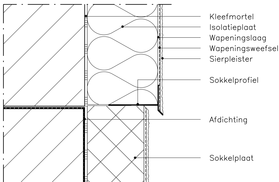
Afb. 32: Thermische onderbroken sokkelprofiel - verticale snede
