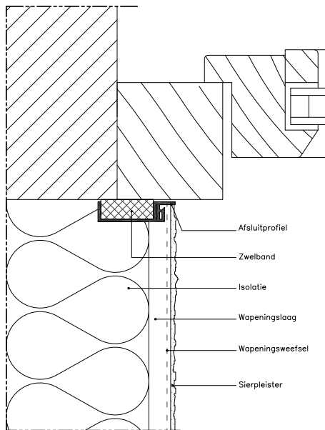
kunststof-profiel (met weefsel)
