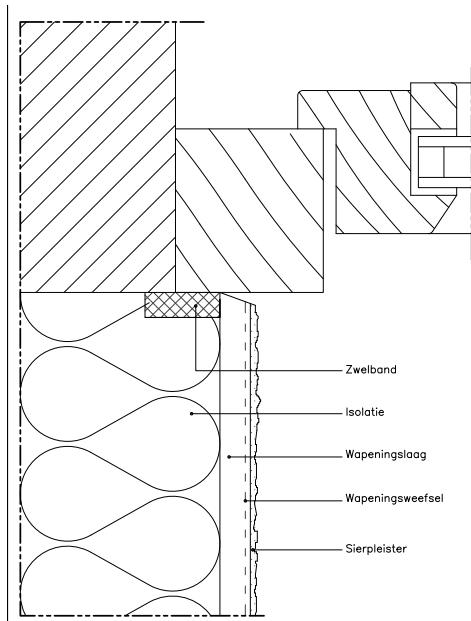
enkel zwelband (met V- groef)
